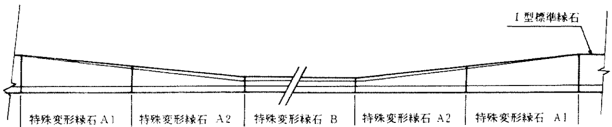
施工图
