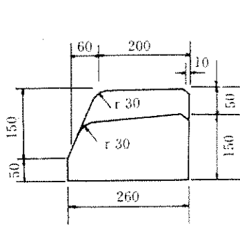
特殊变形 A 2
