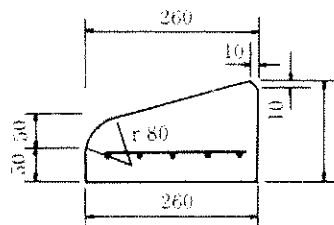
特殊変形 A
