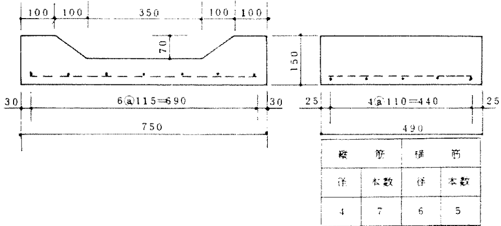
皿型側溝 III 型 (土現規格)
