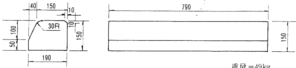
変形 A 150×190×150/100×790mm
