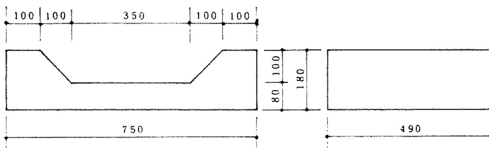
皿型側溝 IV 型 (土現規格)
