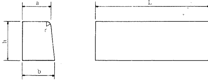
地先境界ブロック
