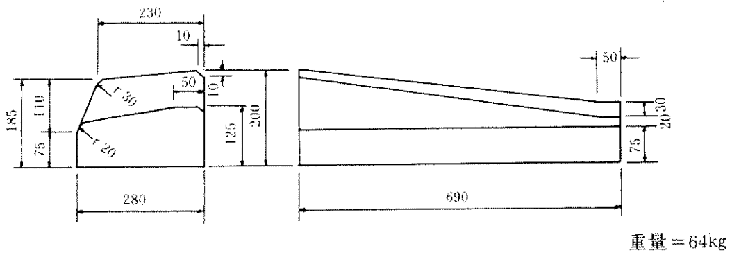
特殊变形 A2
