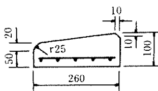
特殊変形 B
