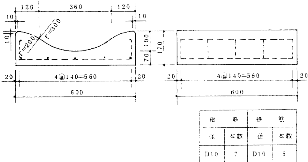
皿型側溝 III 型 (土現規格)
