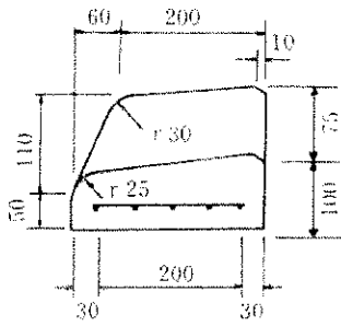
特殊变形 A 2
