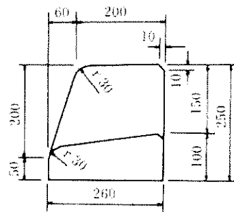
特殊変形 A
