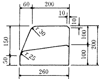
特殊変形 A
