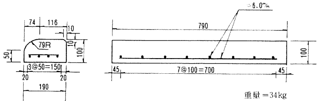
変形 B 190×100×790mm
