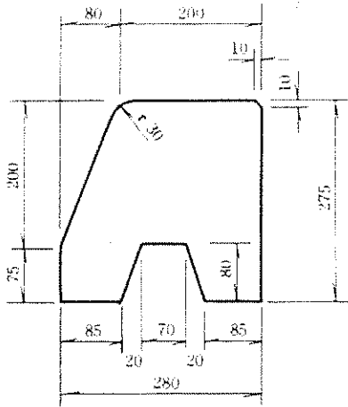
ND-2 標準縁石
